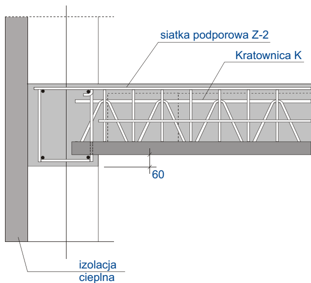
Zasady układania siatek zaginanych Z-2 na ścianach konstrukcyjnych zewnętrznych
